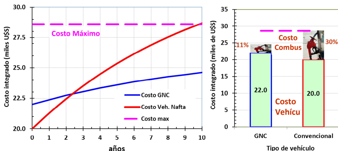
Figura 4. Comparación de los costos y combustible para un vehículo de combustión interna, operando a nafta (convencional) y el equivalente a GNC. A la izquierda se observa que con un uso de 15 000 km/año, a los costos indicados, en 2,3 años se recupera la inversión del equipo de GNC. A la derecha se indica en cada caso el costo del vehículo y combustible usado a lo largo de 10 años, actualizados al valor presente con una TIR=10%. Si el kilometraje recorrido anualmente fuese el doble, el tiempo de recupero se reduce a 1,5 años.
